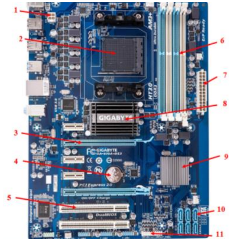
Рисунок 1 – Материнская плата
